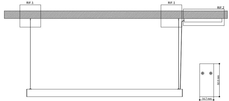
PROSPETTO/FRONT
