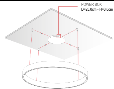
OLIMPIA CON BOX OLIMPIA WITH POWER SUPPLY BOX
