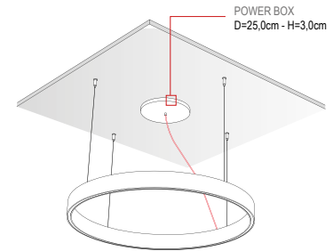
OLIMPIA CON BOX OLIMPIA WITH POWER SUPPLY BOX
